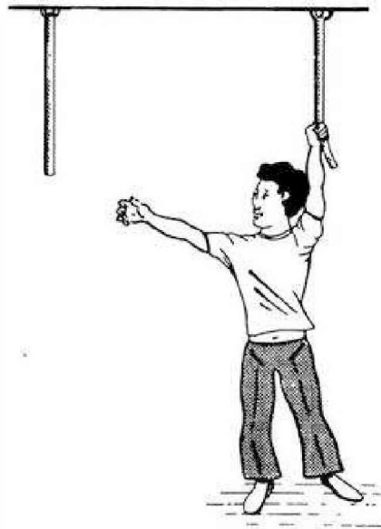
Рис. 9.17. Задача о двух веревках. Как ухватить две веревки одновременно? (Maier, 1930)
